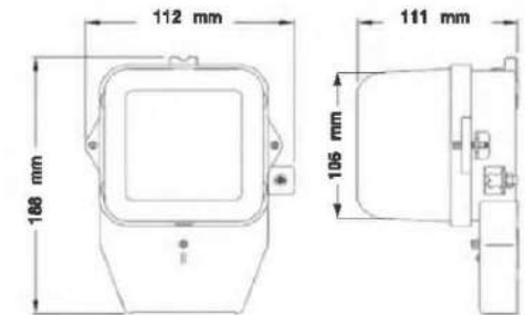
มิติของมิเตอร์ไฟฟ้า
