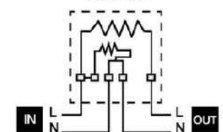
การต่อวงจร
