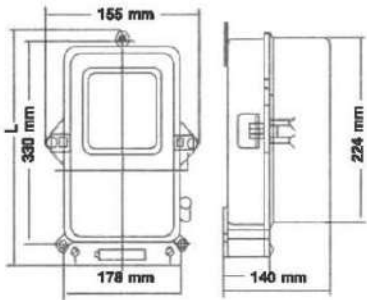
มิติของมิเตอร์ไฟฟ้า
