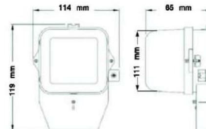
มิติของมิเตอร์ไฟฟ้า
