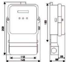
มิติของมิเตอร์ไฟฟ้า
