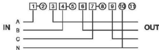
การต่อวงจร
