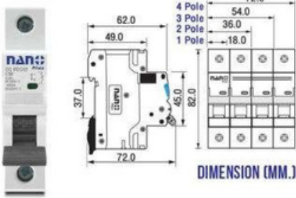
เซอร์กิตเบรกเกอร์ DC (MCB) 1 Pole 10 kA
