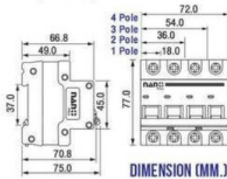
เซอร์กิตเบรกเกอร์ (MCB) 1 Pole 6 kA
